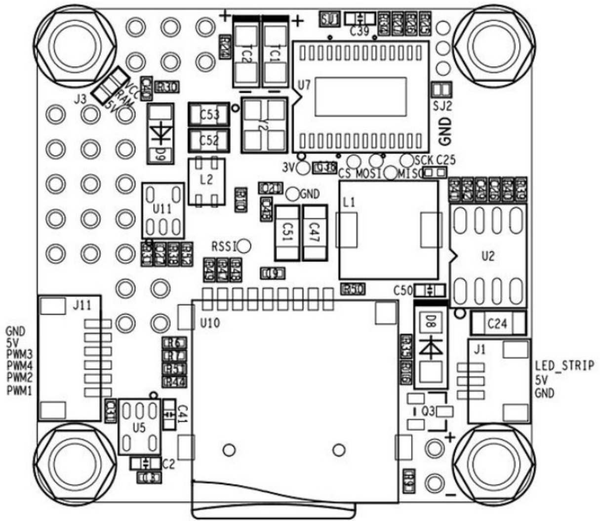
OmnibusF4-Pro-0A
