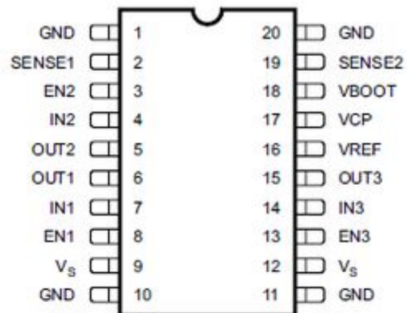
PowerSO20
