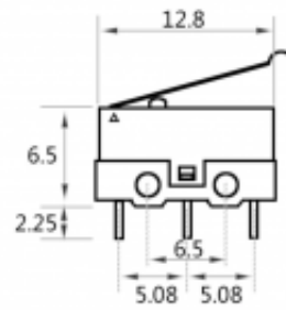
Mini Micro Limit Switch Ultra Small 1A
