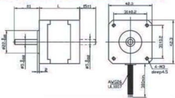
外型图 ( Mechanical Dimensions ) : unit=mm
