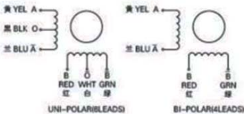
接线图 ( Wiring Diagram ) :
